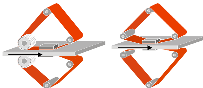
Комбинация: Контактный валок и прижимная балка
